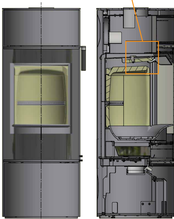
Mocowanie górnej płyty dopalającej
