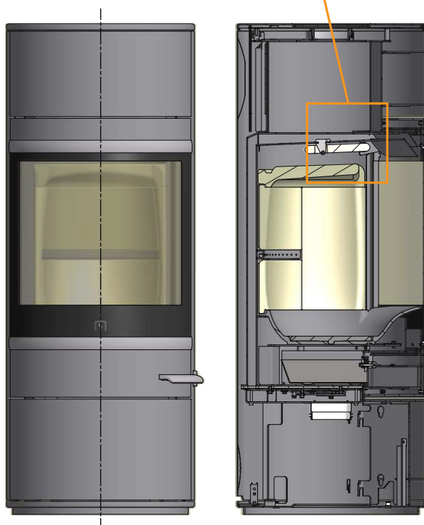
Mocowanie górnej płyty dopalającej
