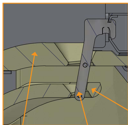
Górna płyta dopalająca
