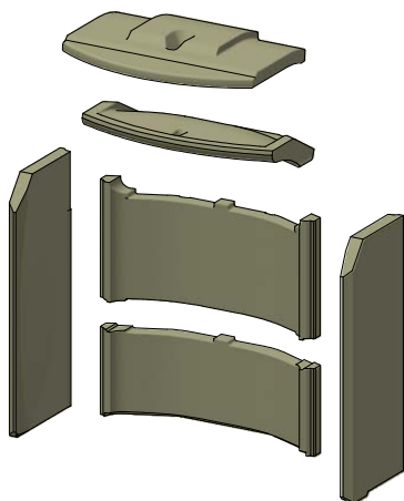
Płyty wewnętrzne komory spalania
