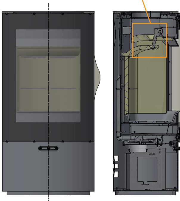
Mocowanie płyt dopalających
