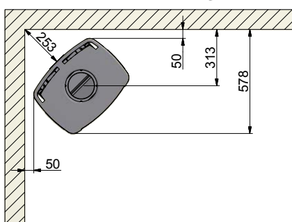
65-1, 65-3, 65-7 i 65-9 (Bez szyb bocznych) Montaż pod kątem 45° w rogu pomieszczenia
