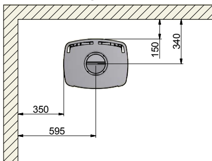
65-1, 65-3, 65-7 i 65-9 (Bez szyb bocznych) Montaż równoległe do ściany
