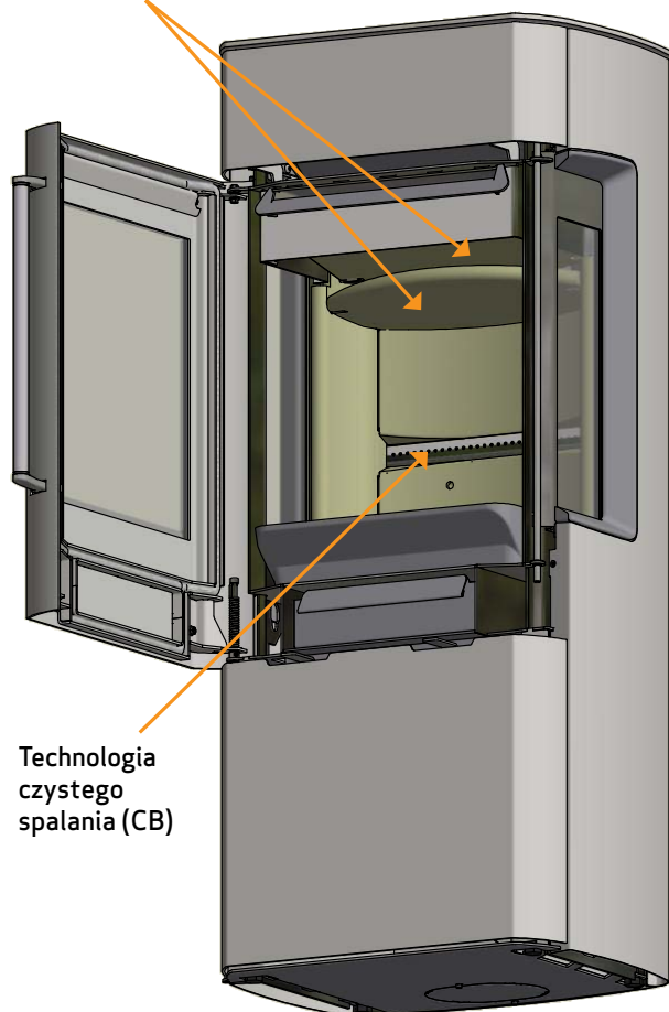
Płyty dopalające
